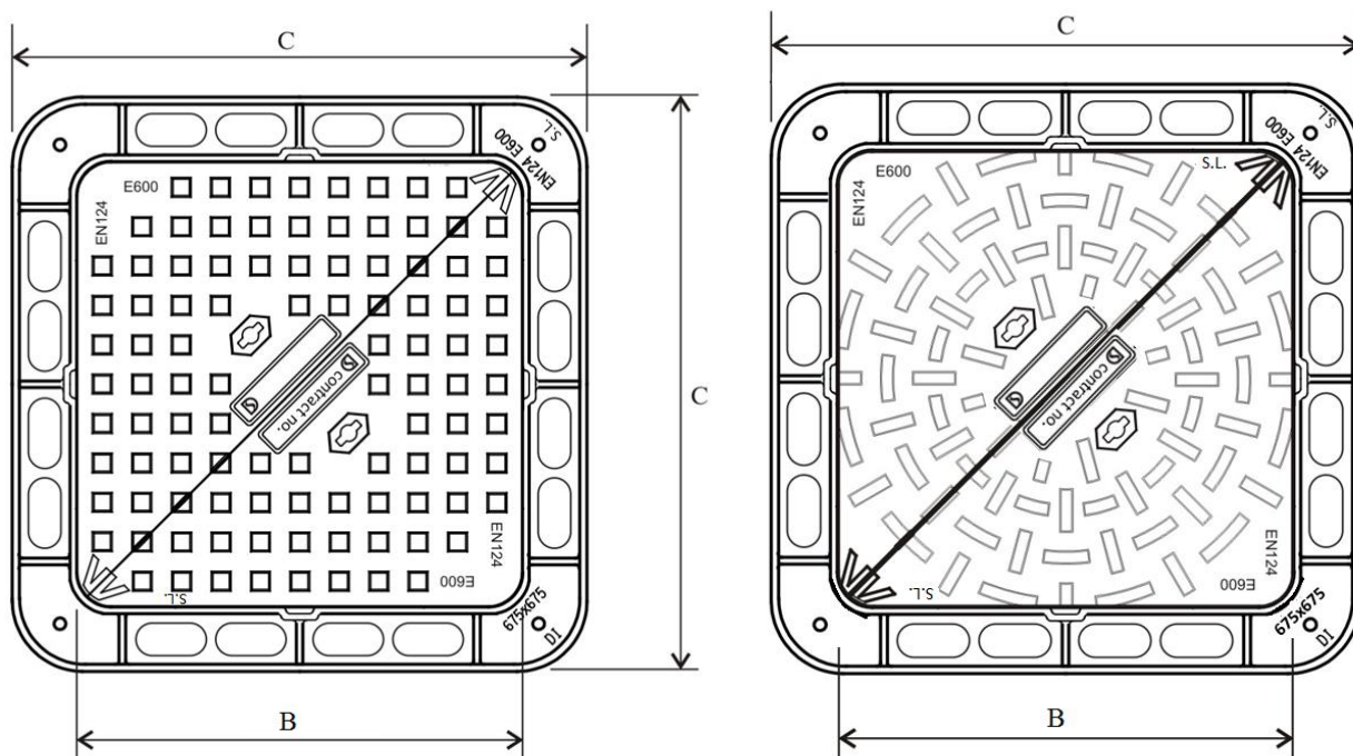
FOUL WATER 污水
