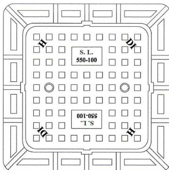
FOUL WATER 污水
